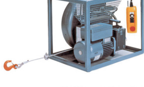
Tirak™ - przenośna wciągarka w obudowie z nawojem liny.
